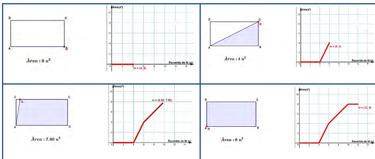
Figura 4. Representación gráfica_ GeoGebra
