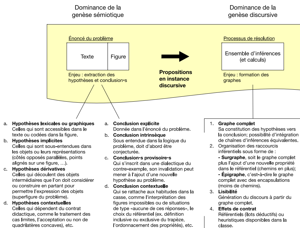
Figure 30. Génèses sémiotiques et discursives dans QED-Tutrix
